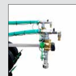
Sistema d'irrigazione a comando elettronico con elettrovalvola con distribuzione sulla pianta
